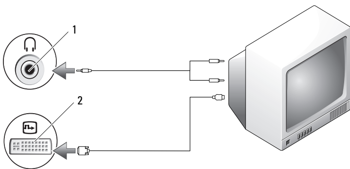
1 音频连接器 2 DVI 连接器
